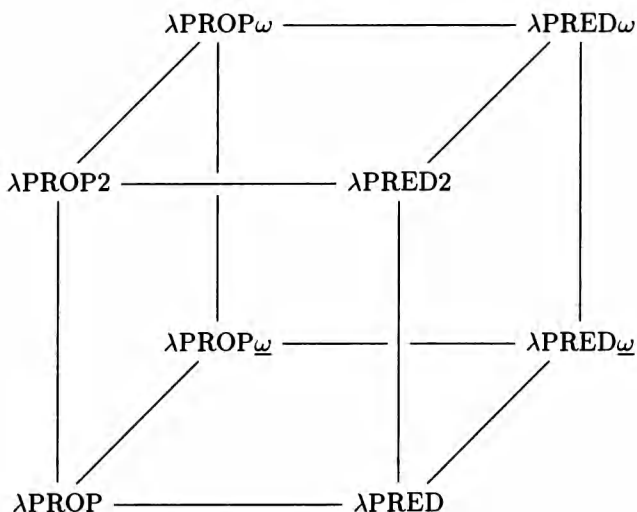
Fig. 4. The L-cube.
